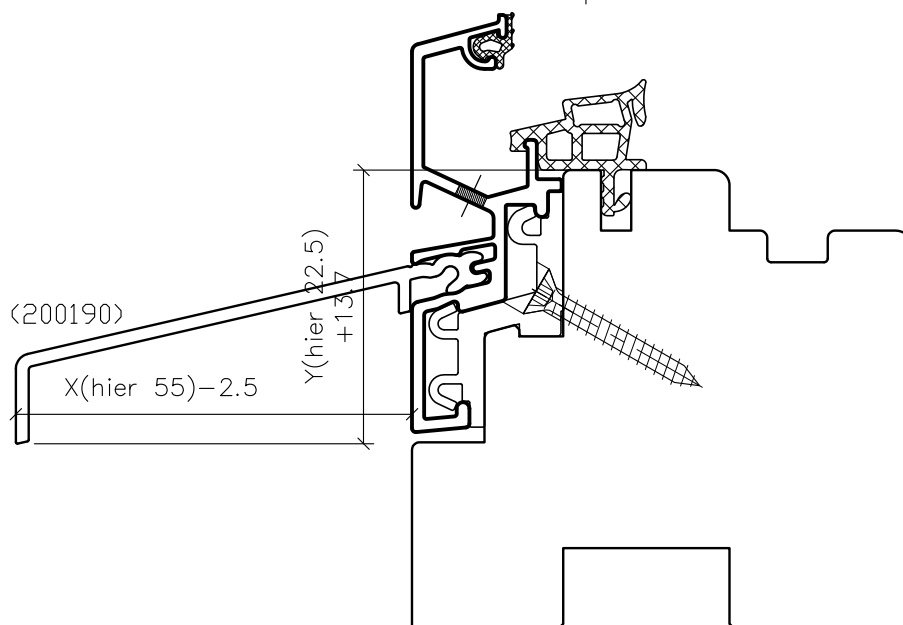
WS-Grundprofil Varia
