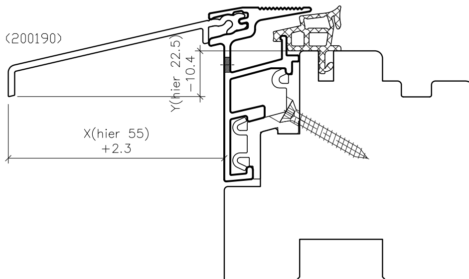
Rollstuhlschwelle Varia
